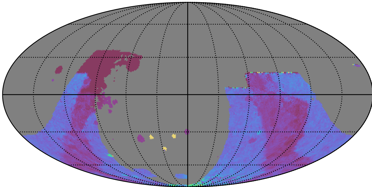
baseline_v3.2_10yrs : GalplaneTimePerFilter_combined_map_u
