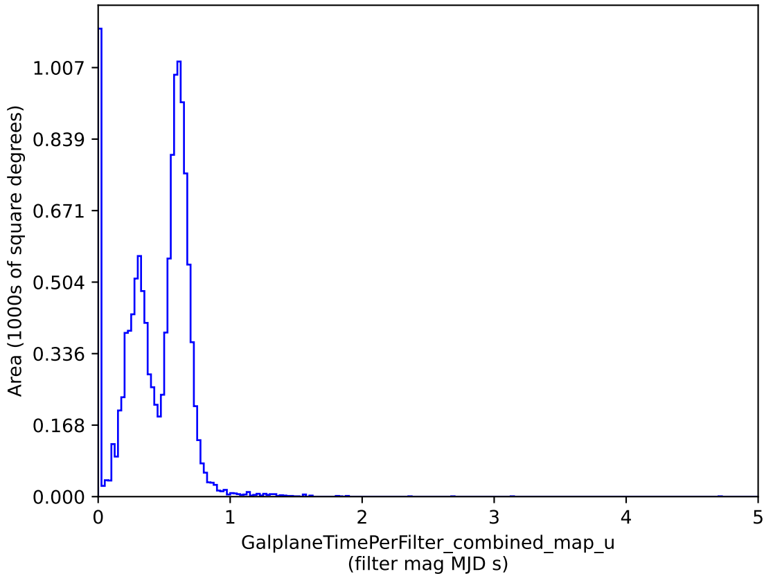
baseline_v3.2_10yrs : GalplaneTimePerFilter_combined_map_u
