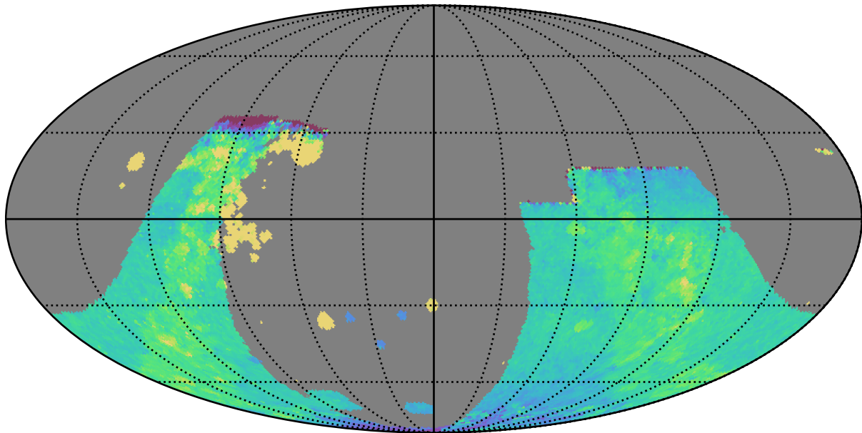
baseline_v3.2_10yrs : GalplaneTimePerFilter_combined_map_i
