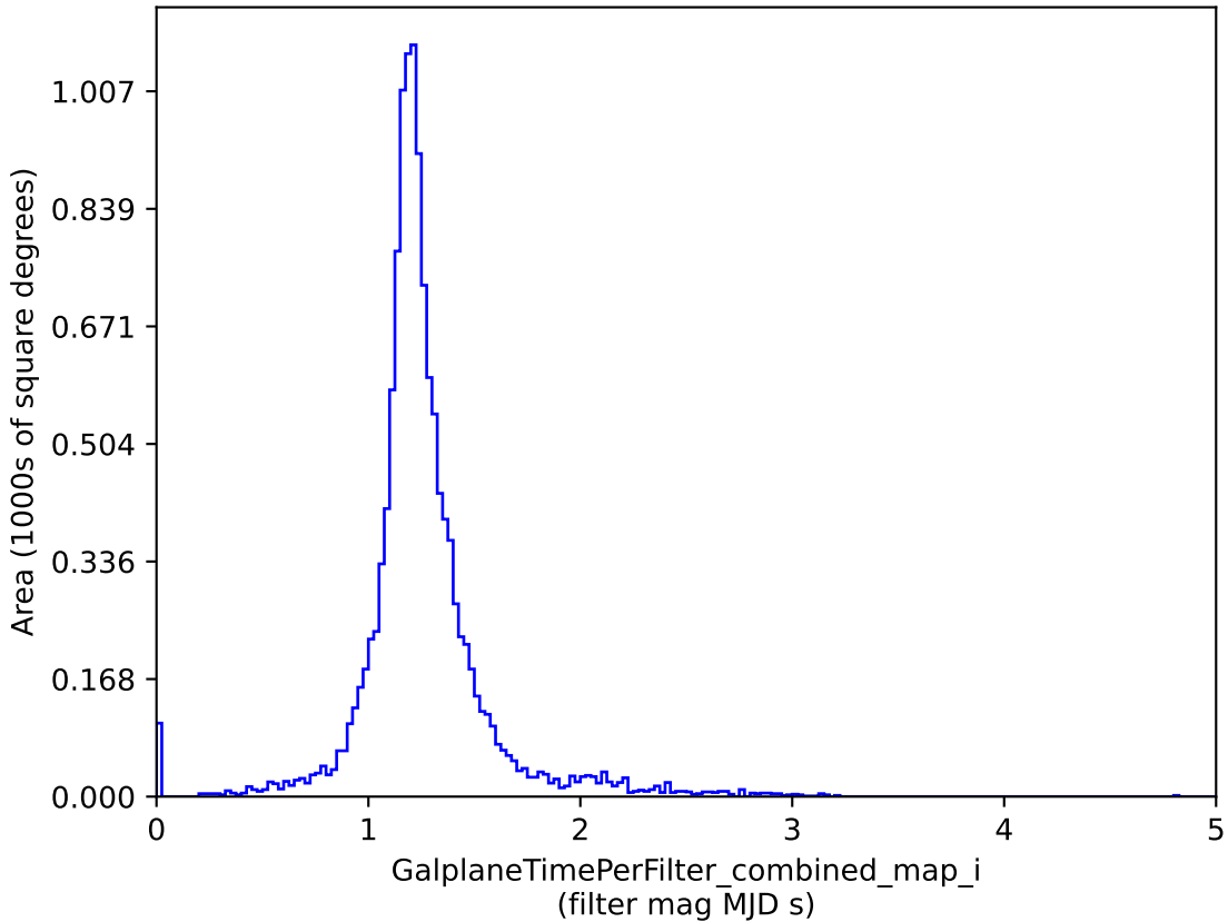
baseline_v3.2_10yrs : GalplaneTimePerFilter_combined_map_i
