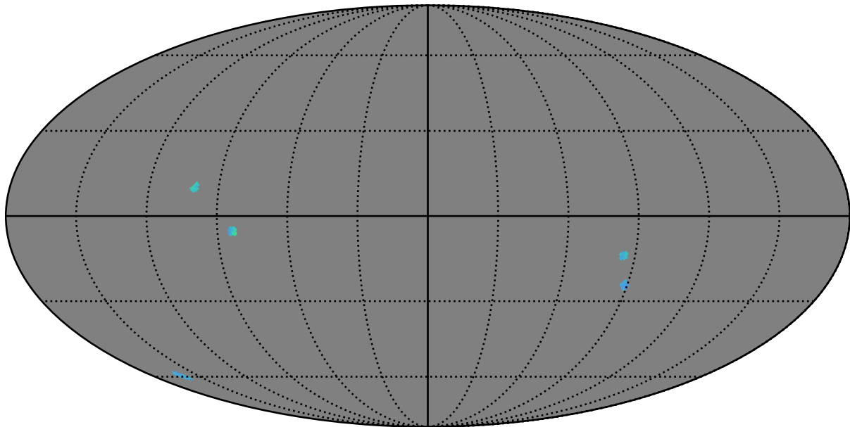
baseline_v3.2_10yrs : GalplaneTimePerFilter_bonito_sfr_map_y
