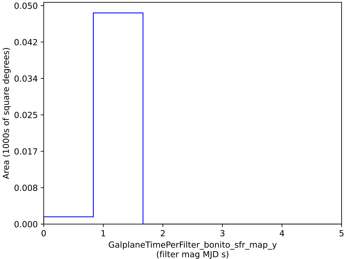
baseline_v3.2_10yrs : GalplaneTimePerFilter_bonito_sfr_map_y
