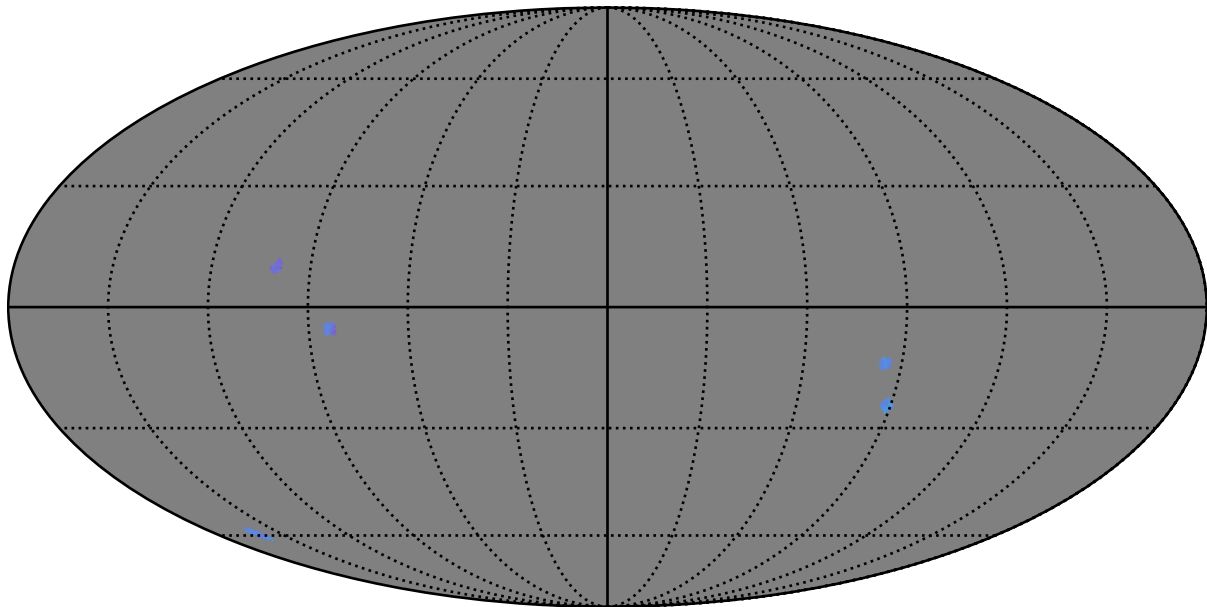
baseline_v3.2_10yrs : GalplaneTimePerFilter_bonito_sfr_map_g
