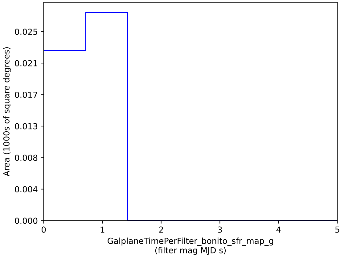
baseline_v3.2_10yrs : GalplaneTimePerFilter_bonito_sfr_map_g
