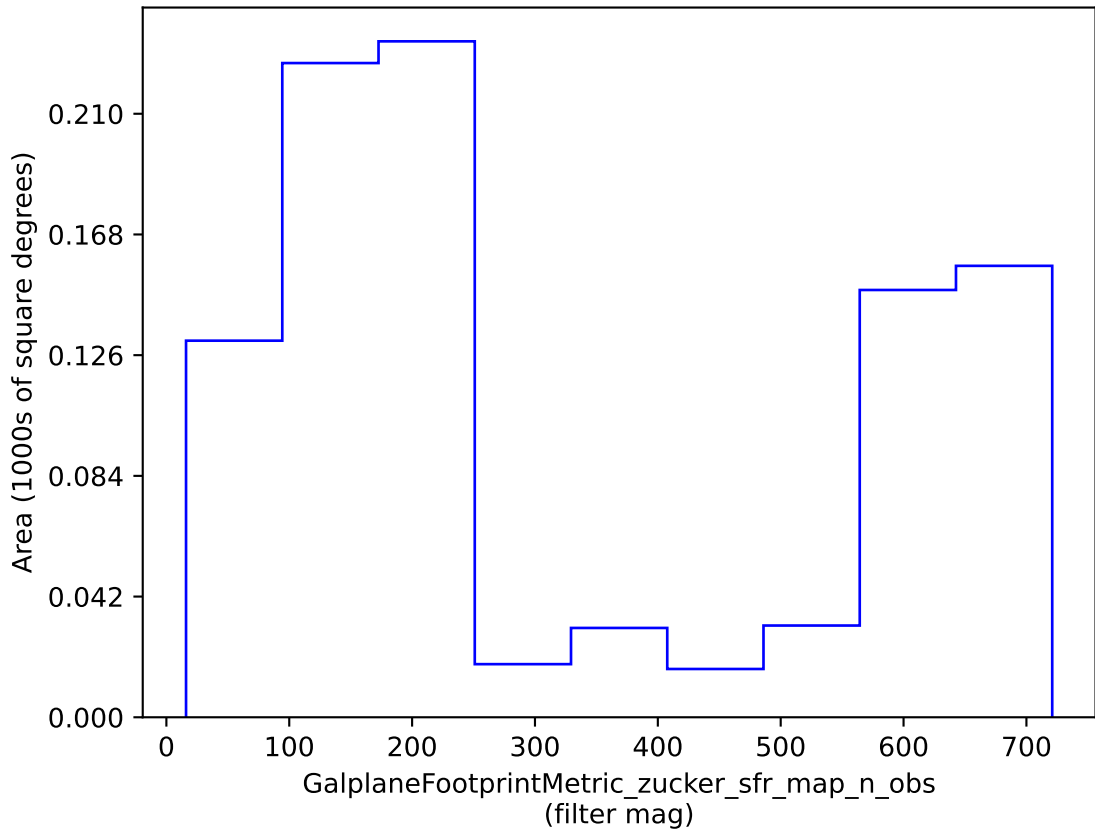
baseline_v3.2_10yrs : GalplaneFootprintMetric_zucker_sfr_map_n_obs
