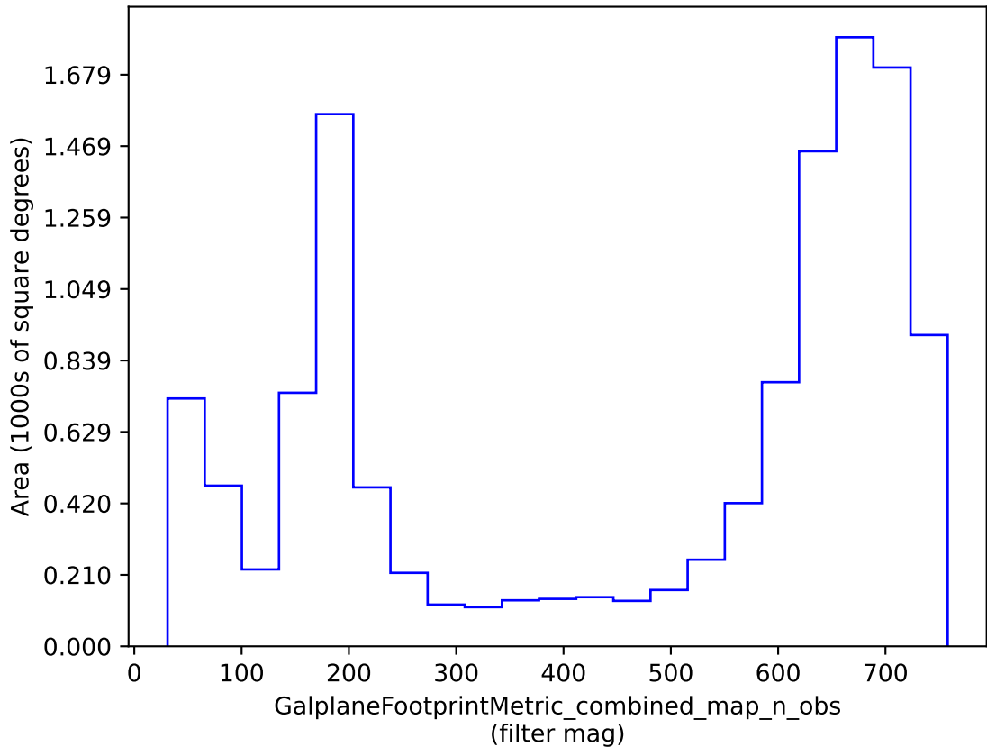
baseline_v3.2_10yrs : GalplaneFootprintMetric_combined_map_n_obs
