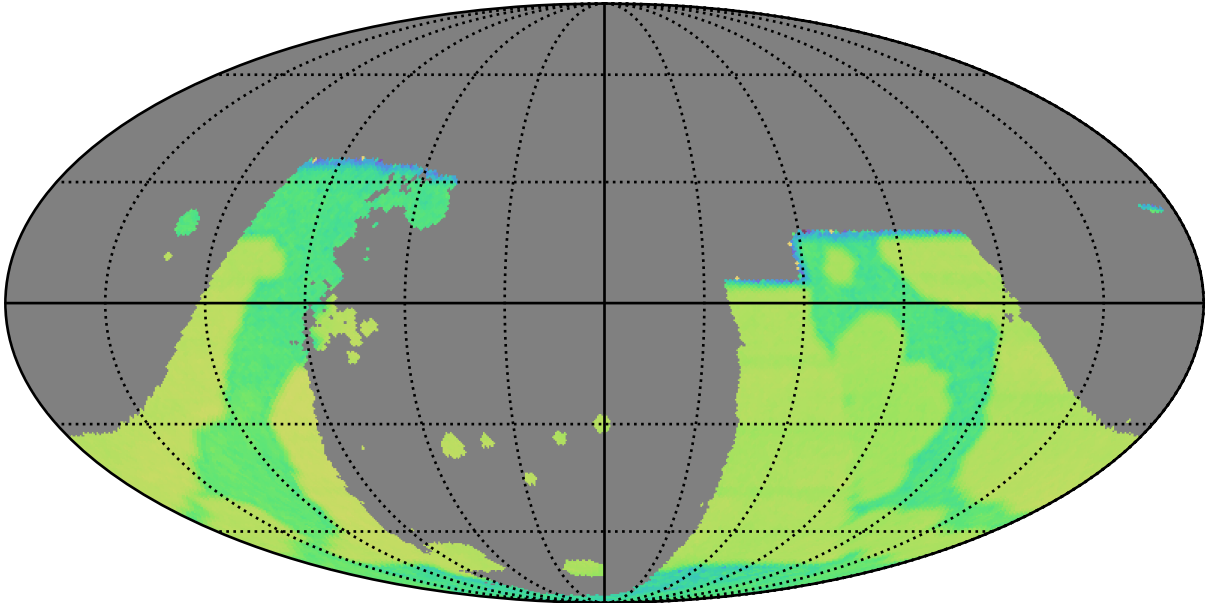
baseline_v3.2_10yrs : GalPlaneVisitIntervalsTimescales_combined_map_Tau_5_0
