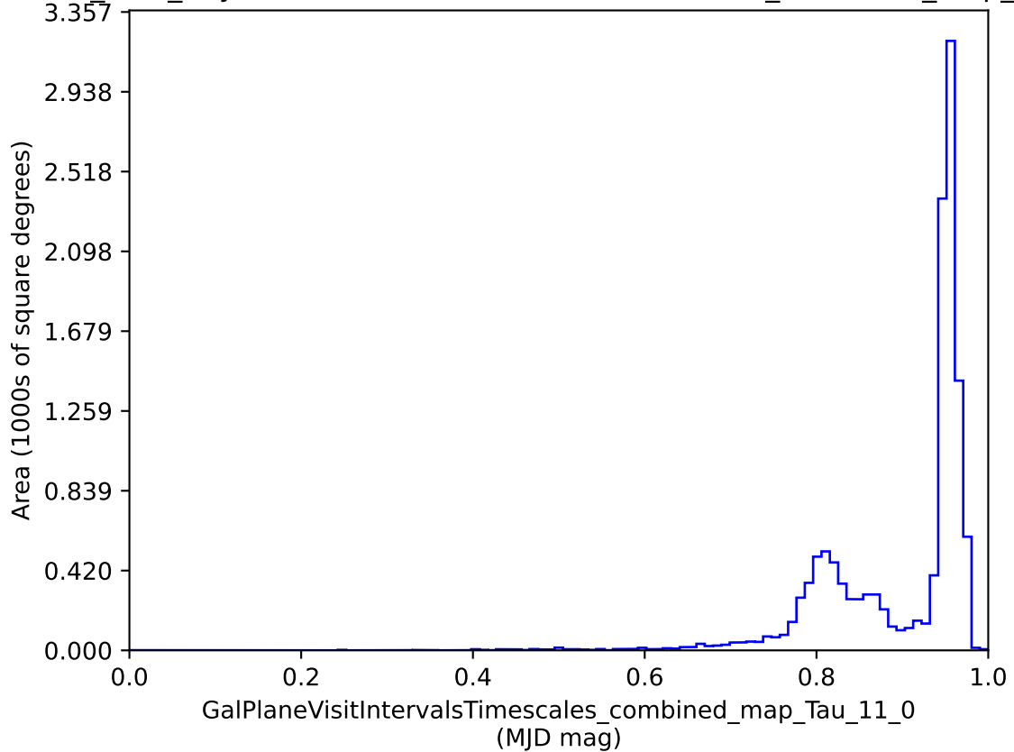
baseline_v3.2_10yrs : GalPlaneVisitIntervalsTimescales_combined_map_Tau_11_0
