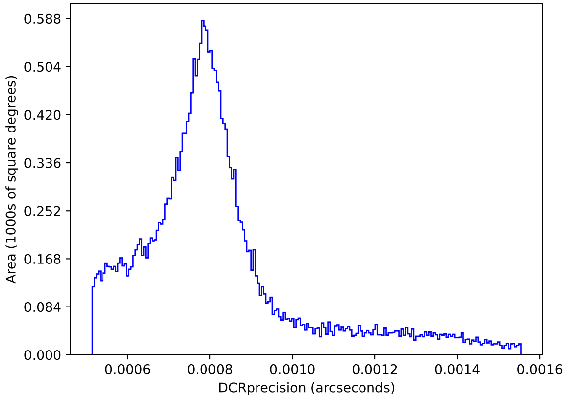
baseline_v3.2_10yrs : DCRprecision
