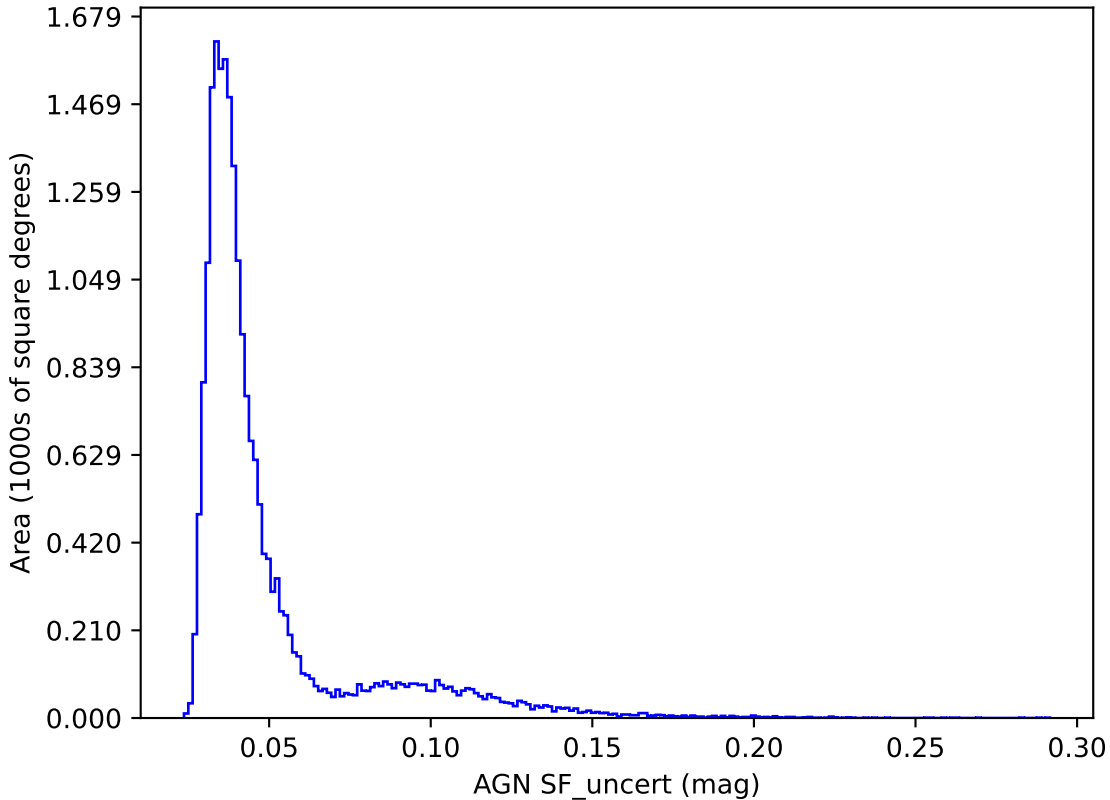
baseline_v3.2_10yrs y band: AGN SF_uncert
