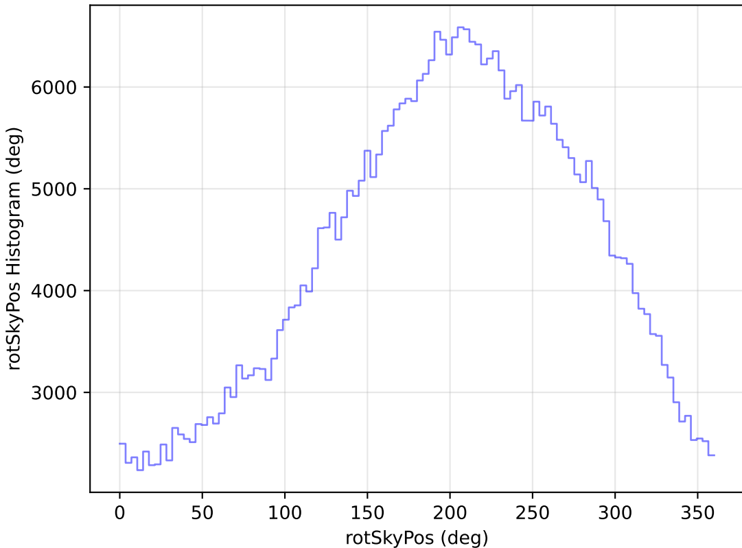
baseline_v3.2_10yrs All sky z band: rotSkyPos Histogram
