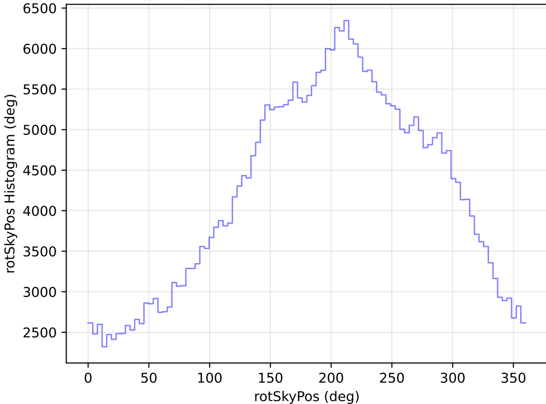
baseline_v3.2_10yrs All sky y band: rotSkyPos Histogram
