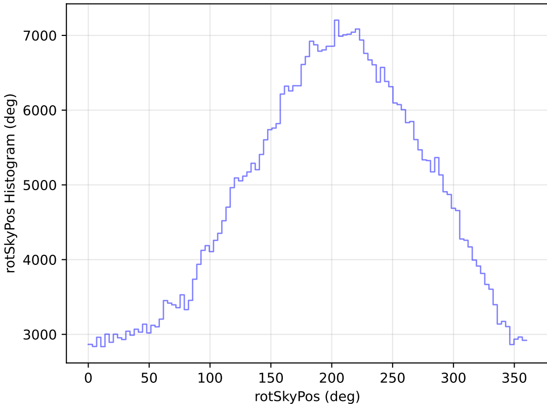
baseline_v3.2_10yrs All sky i band: rotSkyPos Histogram
