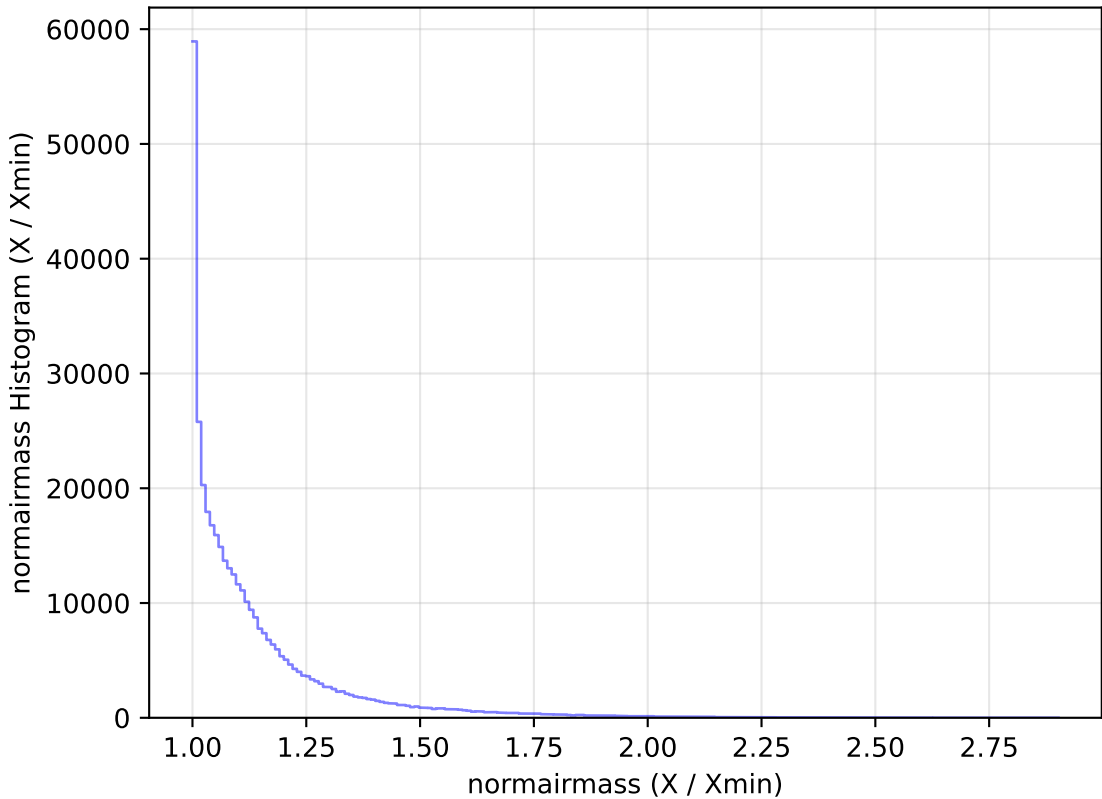
baseline_v3.2_10yrs All sky y band: normairmass Histogram
