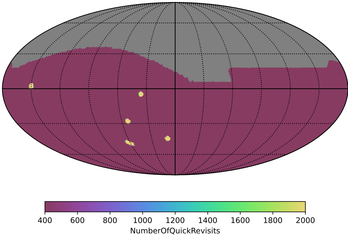
baseline_v3.2_10yrs All sky: NumberOfQuickRevisits
