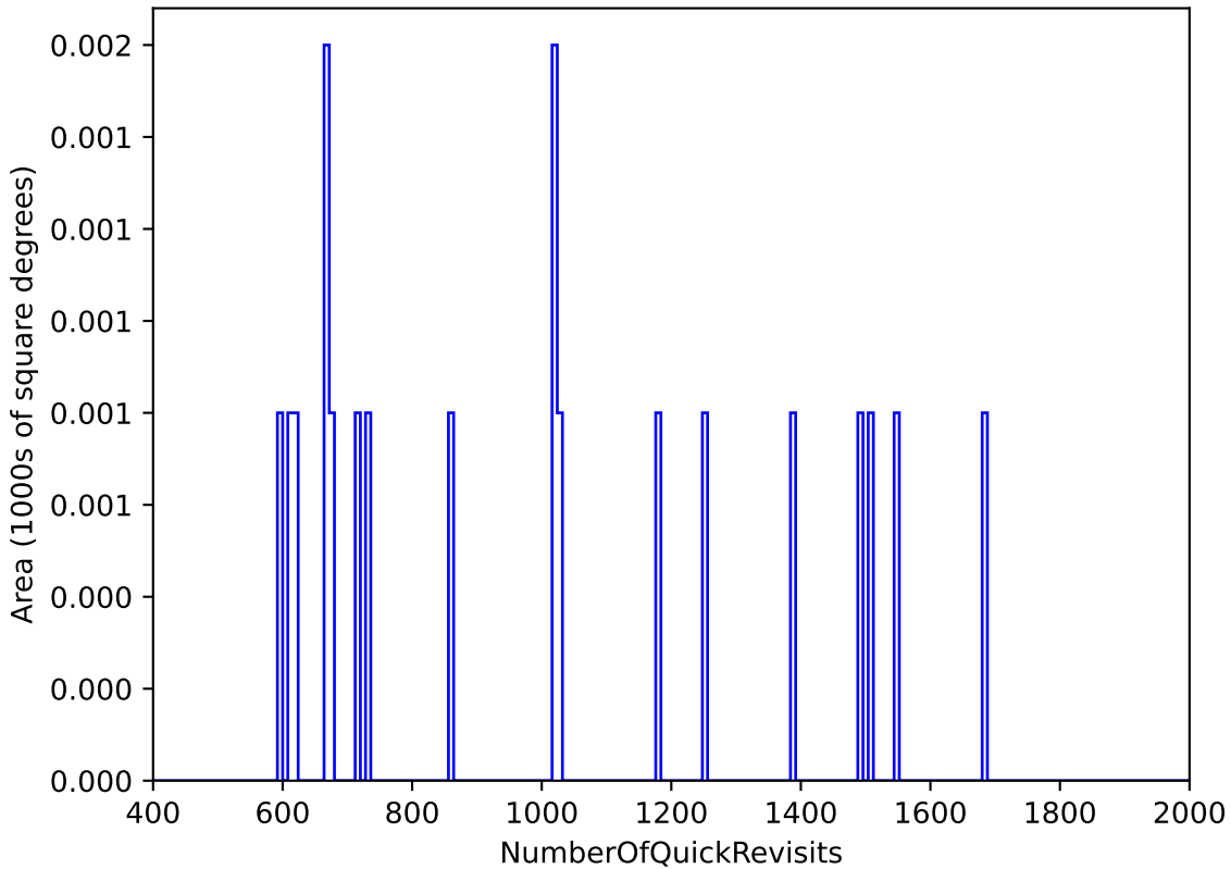
baseline_v3.2_10yrs All sky: NumberOfQuickRevisits
