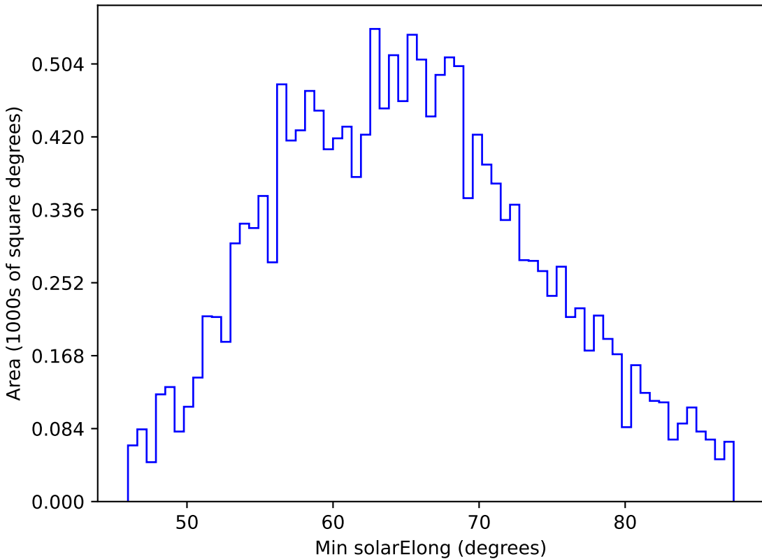
baseline_v3.2_10yrs WFD y band: Min solarElong
