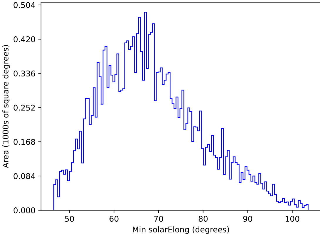
baseline_v3.2_10yrs All sky y band: Min solarElong
