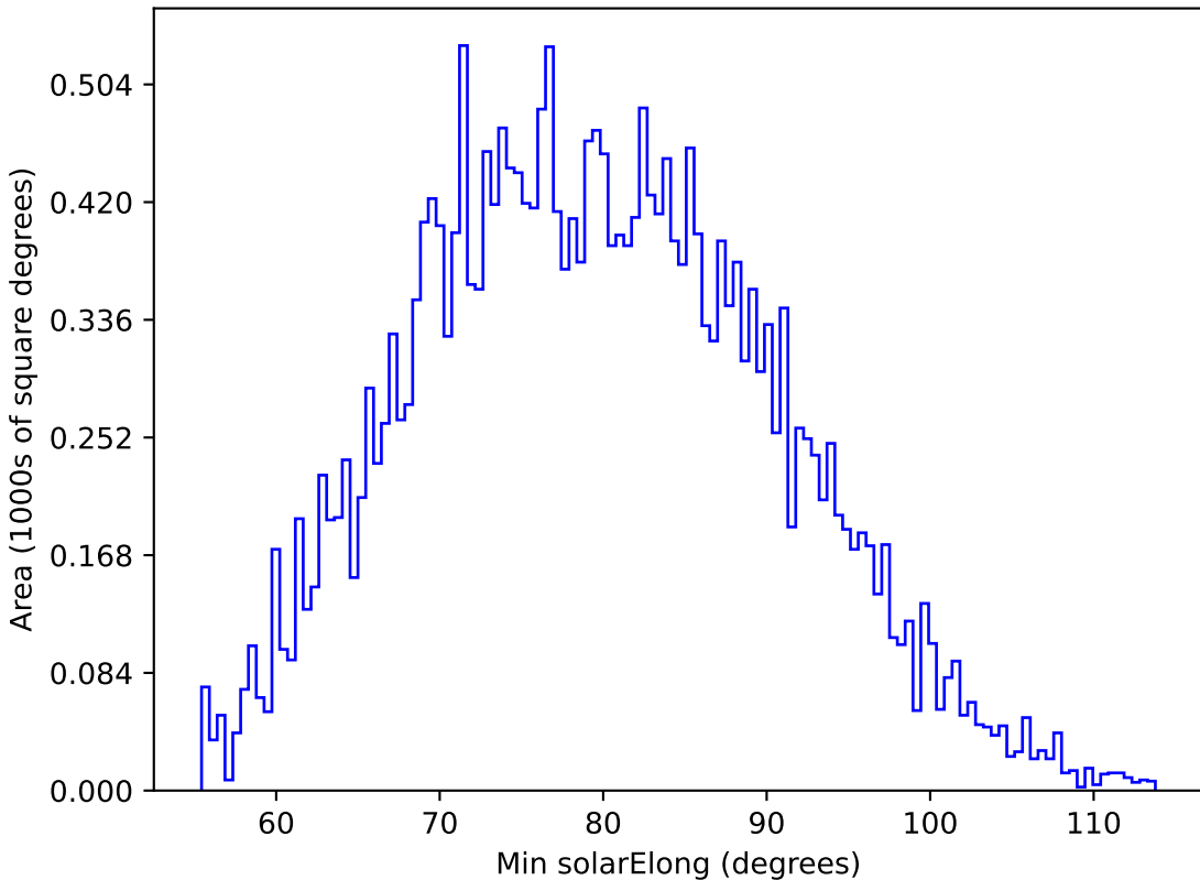
baseline_v3.2_10yrs All sky g band: Min solarElong
