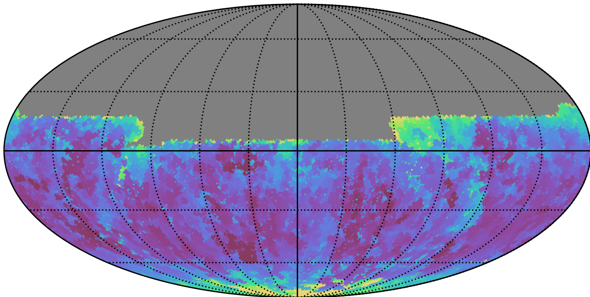
baseline_v3.2_10yrs Yr 1 y band: Min seeingGeom
