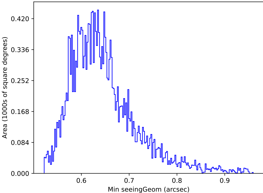
baseline_v3.2_10yrs Yr 1 y band: Min seeingGeom
