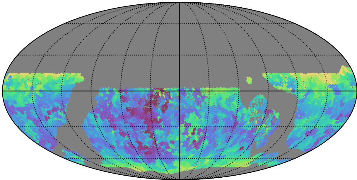
baseline_v3.2_10yrs WFD y band: Min seeingEff
