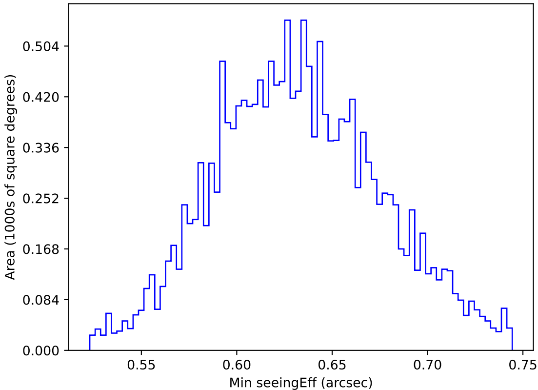
baseline_v3.2_10yrs WFD y band: Min seeingEff
