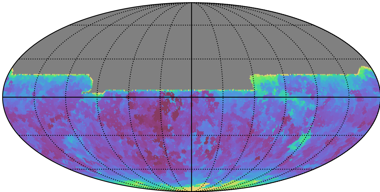
baseline_v3.2_10yrs All sky y band: Min seeingEff
