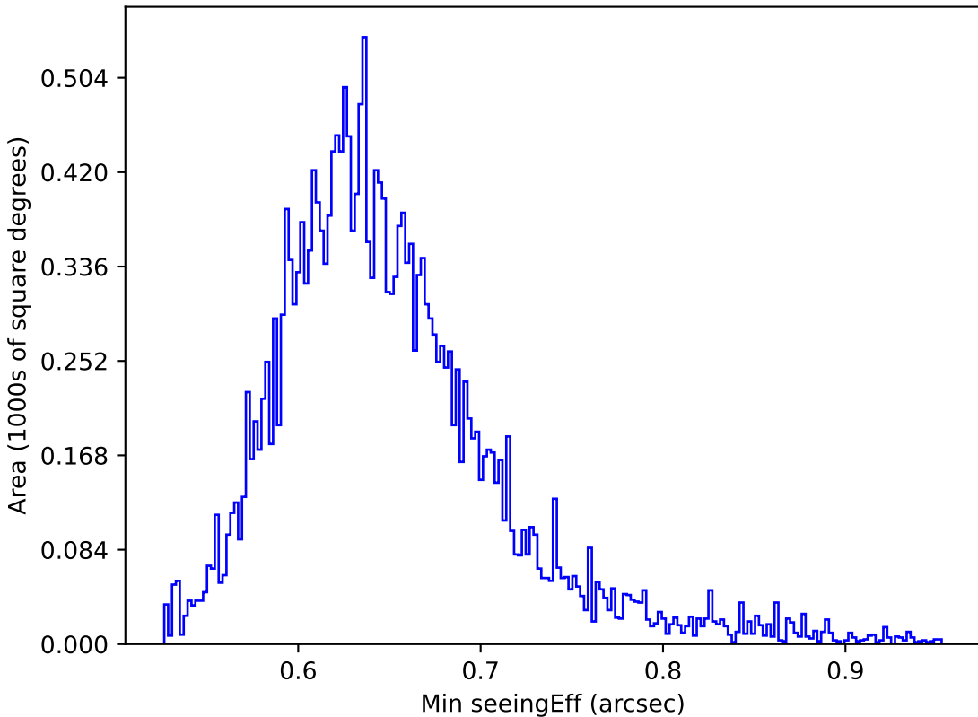
baseline_v3.2_10yrs All sky y band: Min seeingEff
