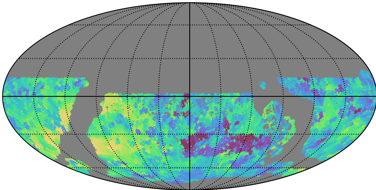
baseline_v3.2_10yrs WFD y band: Min saturation_mag
