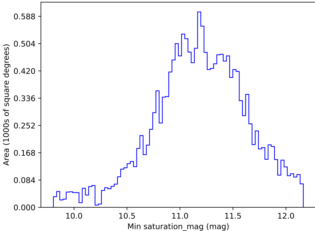
baseline_v3.2_10yrs WFD y band: Min saturation_mag
