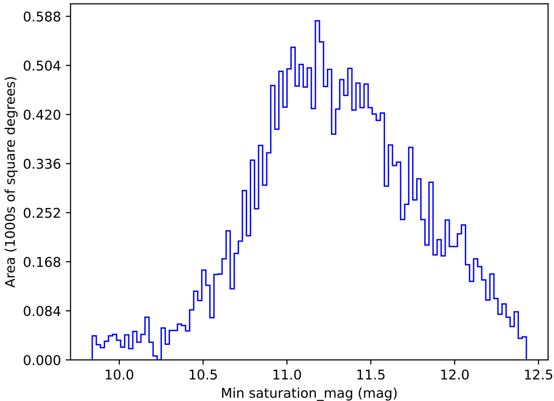
baseline_v3.2_10yrs All sky y band: Min saturation_mag
