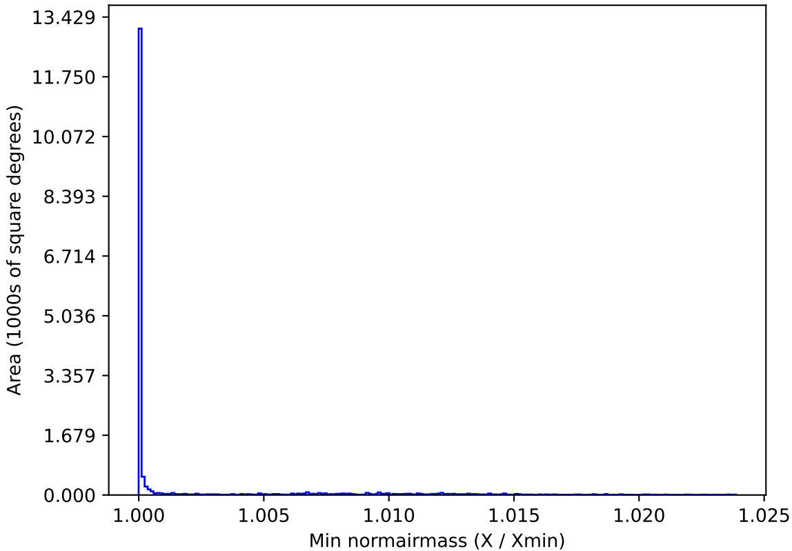
baseline_v3.2_10yrs WFD z band: Min normairmass
