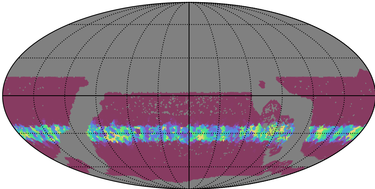
baseline_v3.2_10yrs WFD y band: Min normairmass
