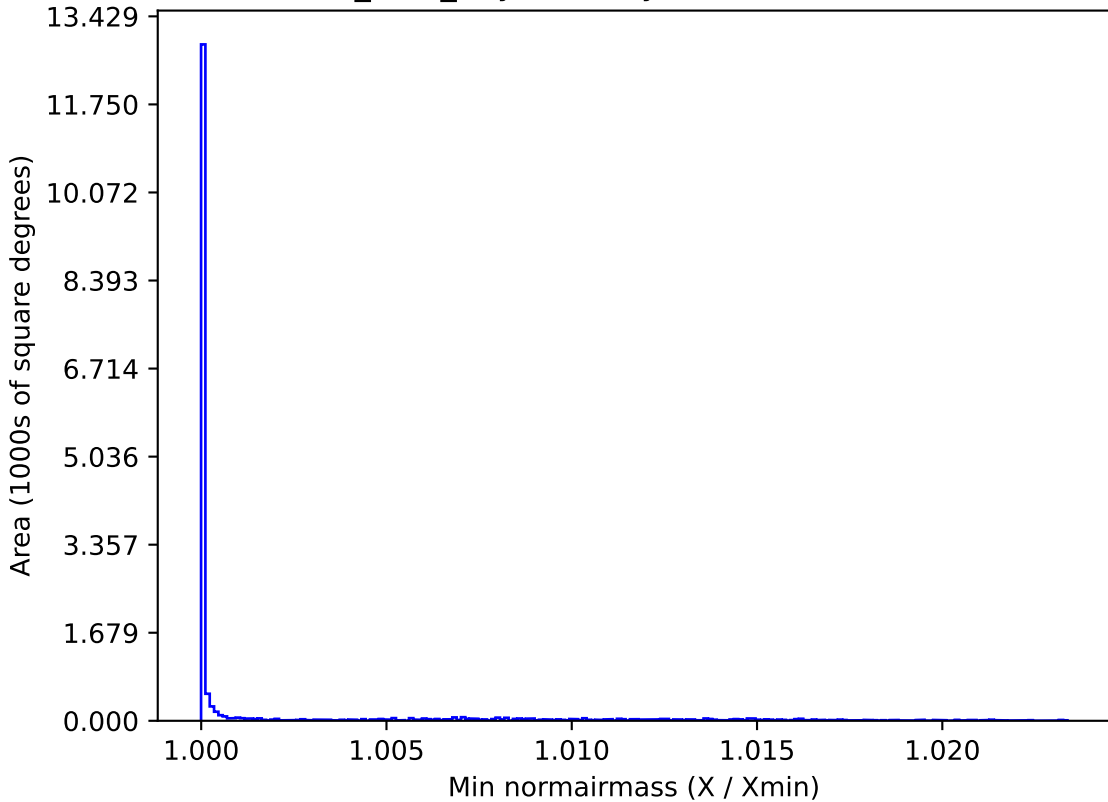
baseline_v3.2_10yrs WFD y band: Min normairmass
