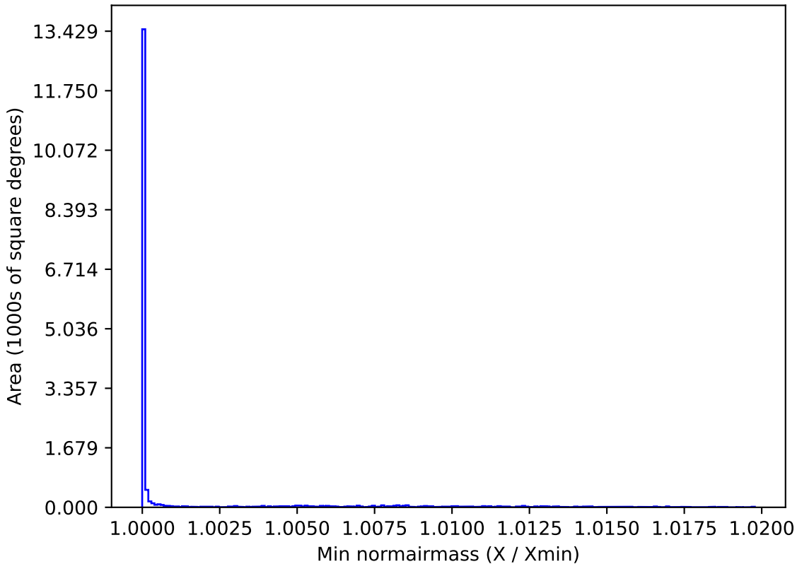
baseline_v3.2_10yrs WFD i band: Min normairmass
