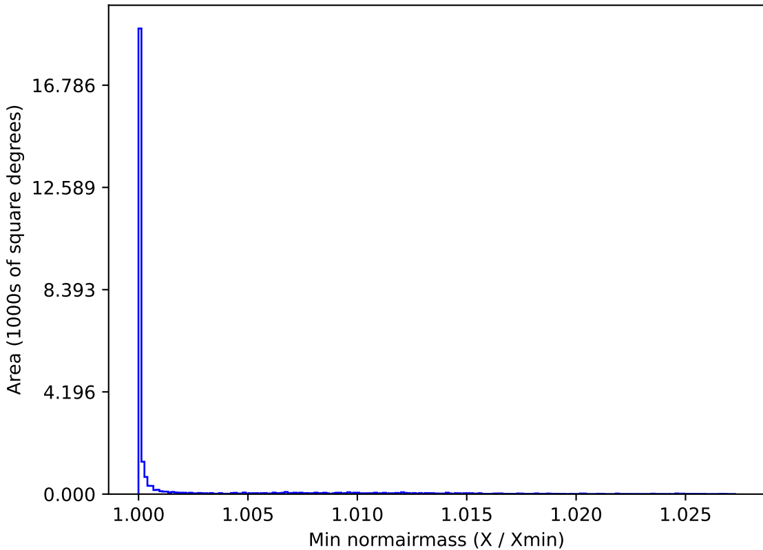
baseline_v3.2_10yrs All sky z band: Min normairmass
