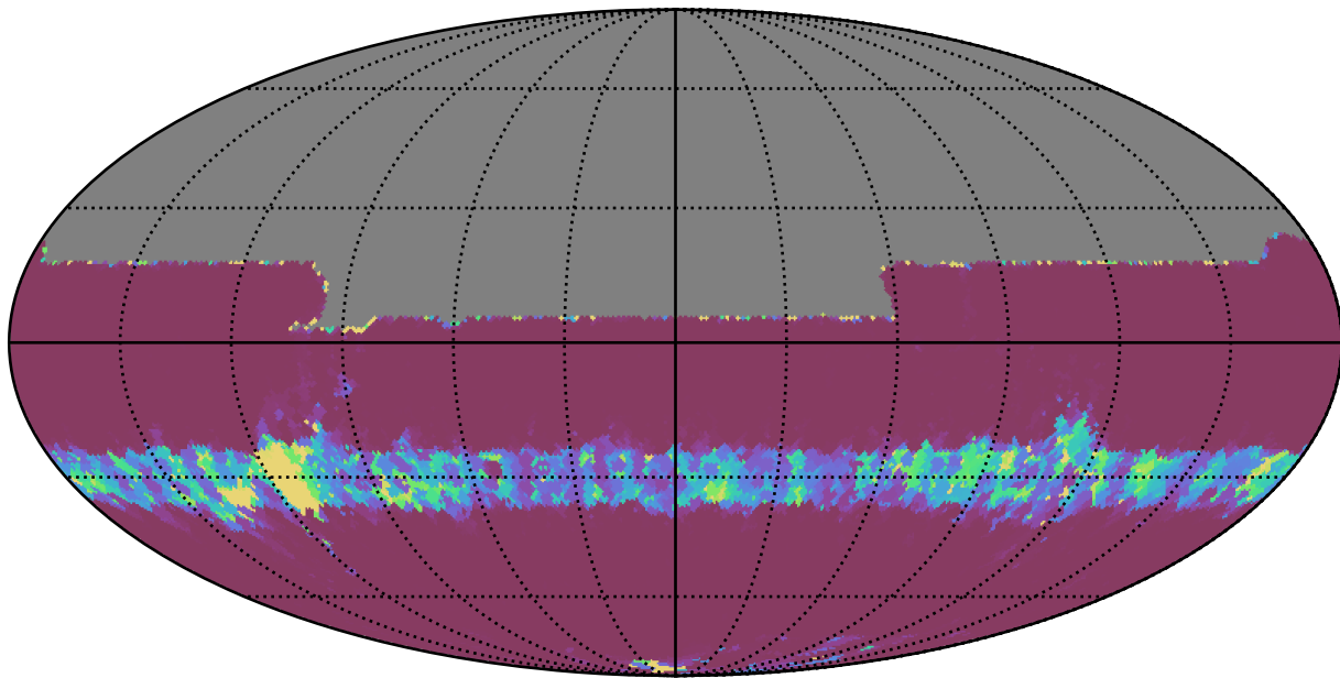
baseline_v3.2_10yrs All sky y band: Min normairmass
