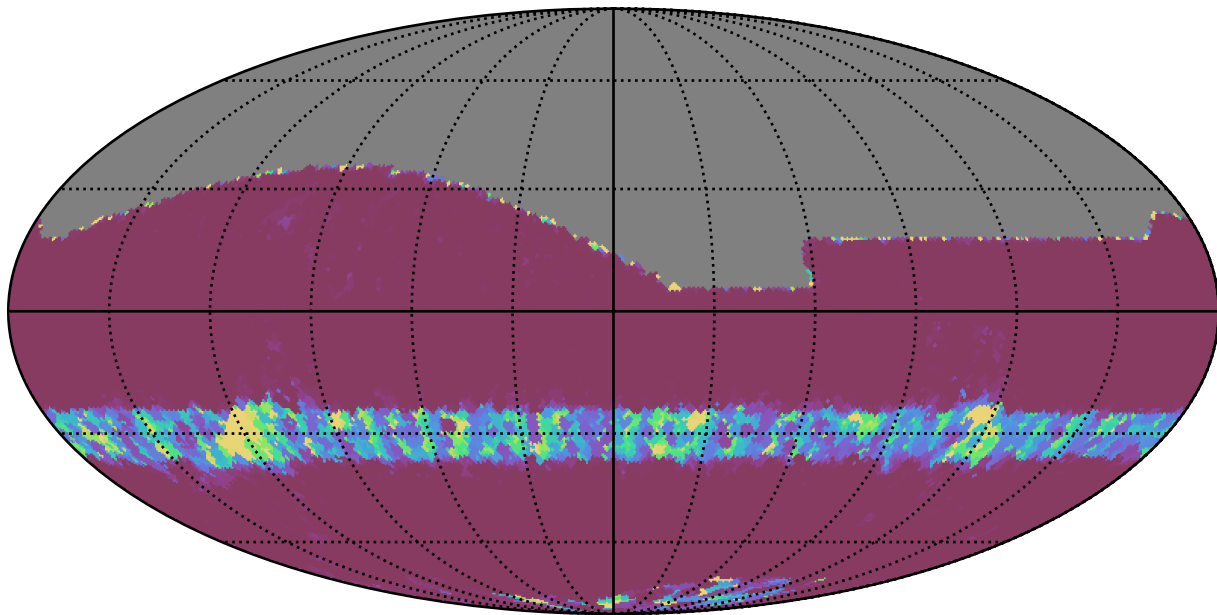
baseline_v3.2_10yrs All sky r band: Min normairmass
