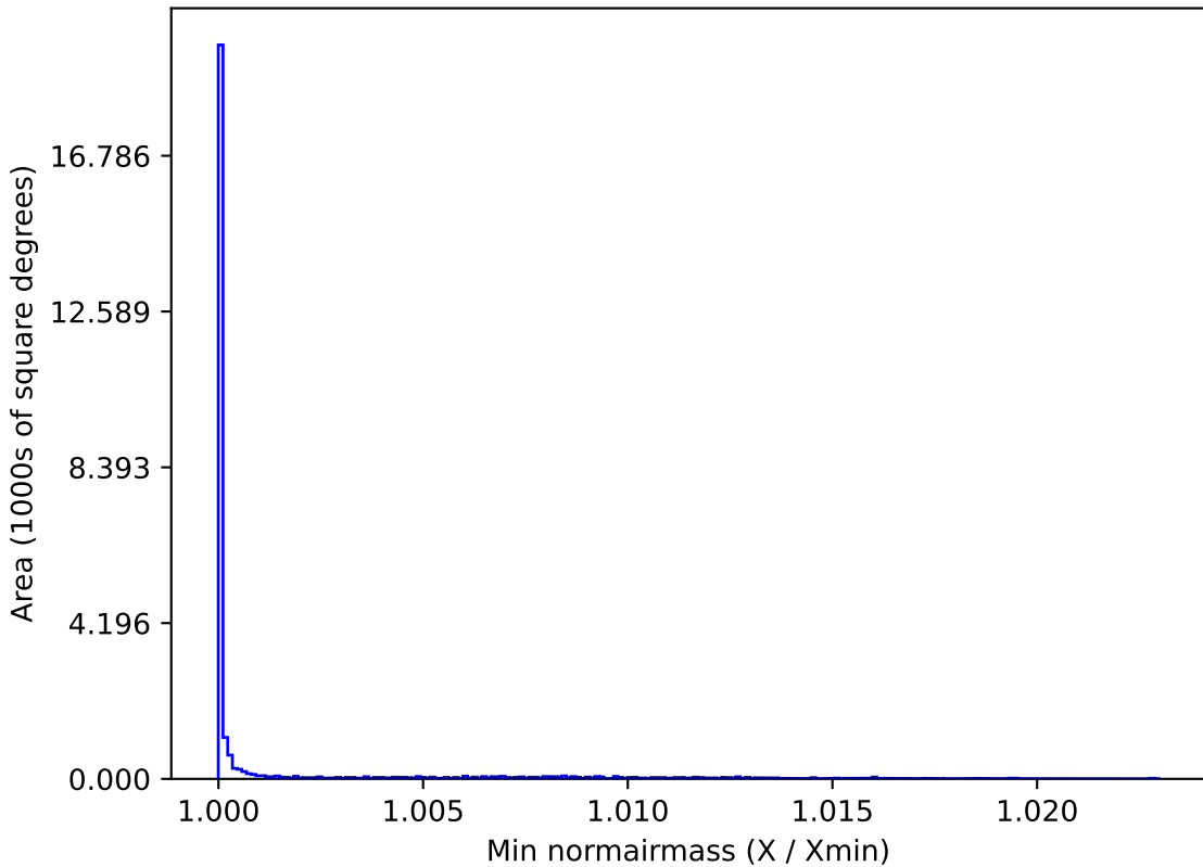
baseline_v3.2_10yrs All sky r band: Min normairmass
