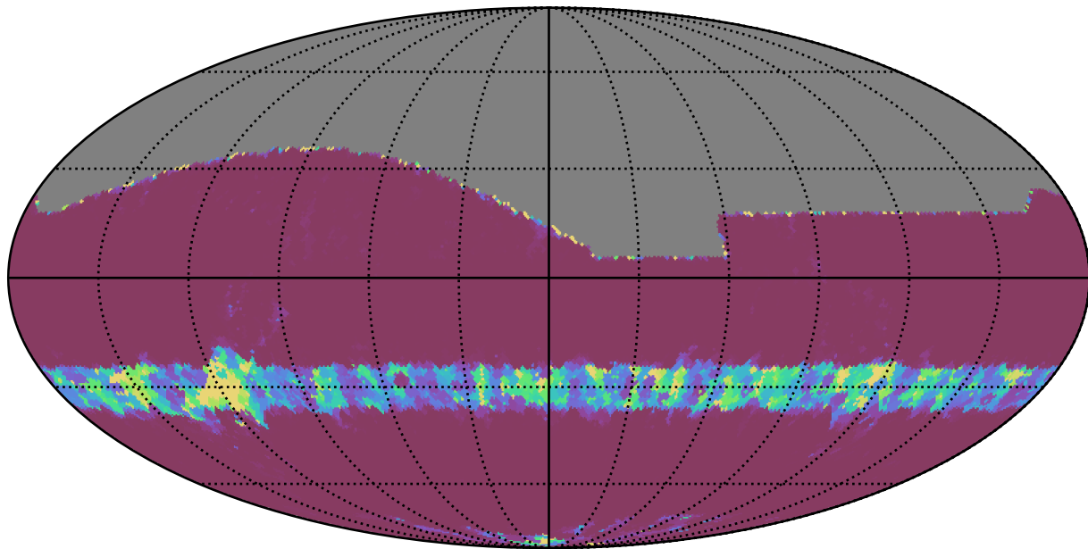
baseline_v3.2_10yrs All sky i band: Min normairmass
