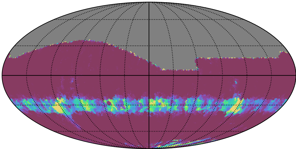
baseline_v3.2_10yrs All sky g band: Min normairmass
