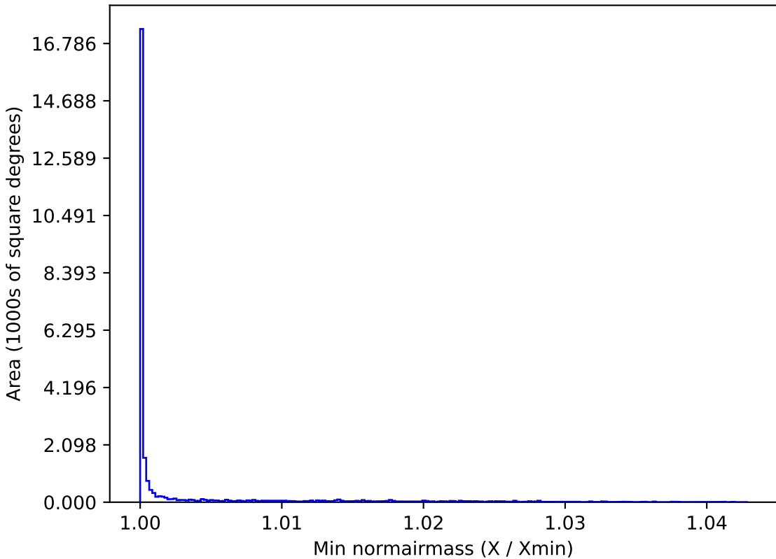
baseline_v3.2_10yrs All sky g band: Min normairmass
