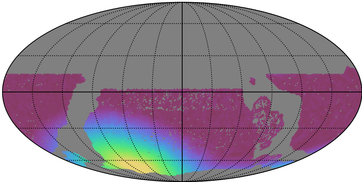
baseline_v3.2_10yrs WFD y band: Min moonDistance
