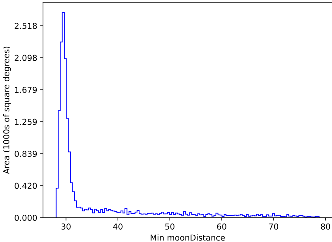
baseline_v3.2_10yrs WFD y band: Min moonDistance
