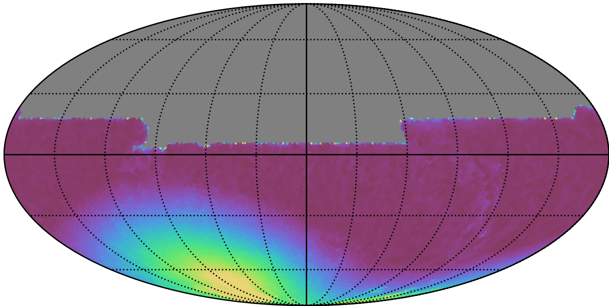
baseline_v3.2_10yrs All sky y band: Min moonDistance
