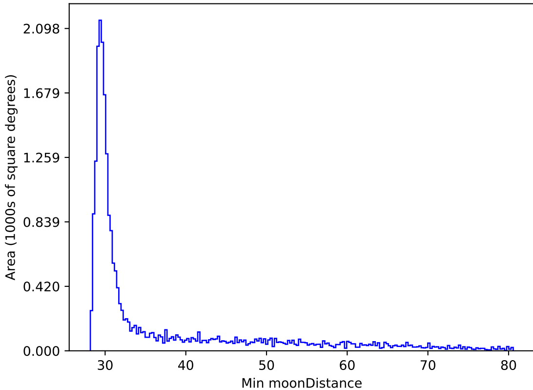
baseline_v3.2_10yrs All sky y band: Min moonDistance
