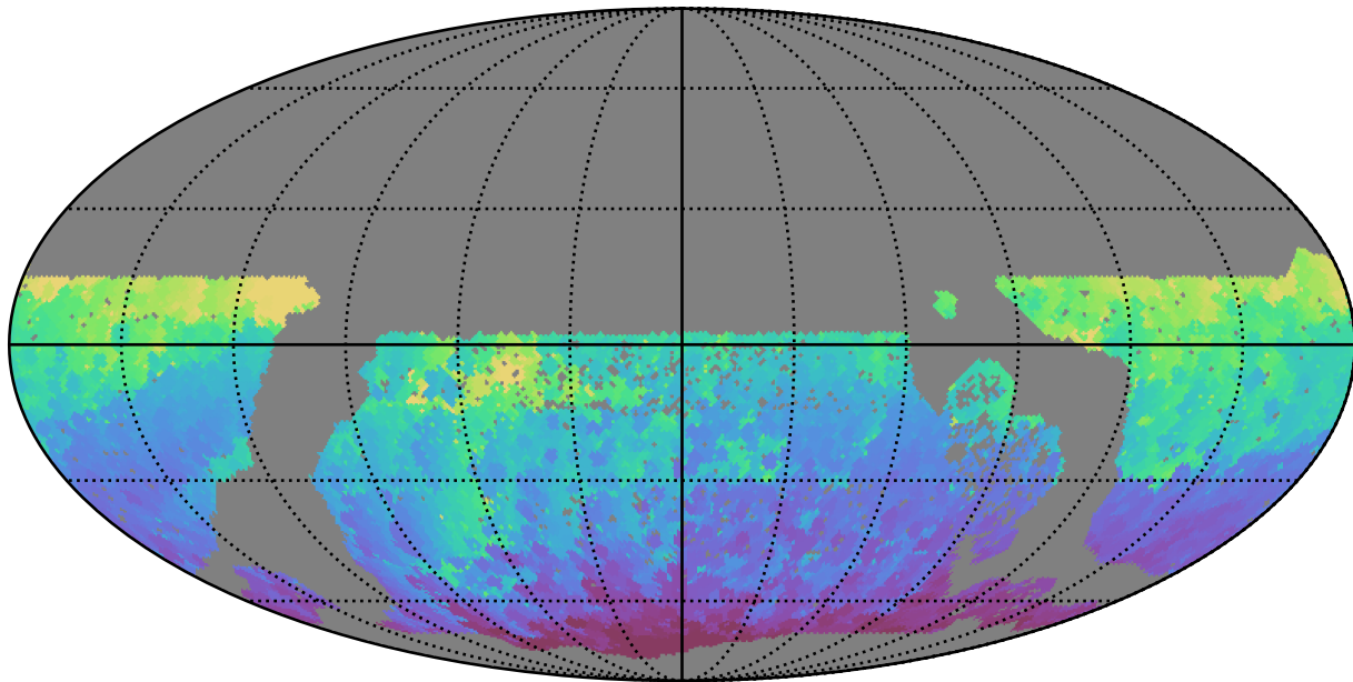
baseline_v3.2_10yrs WFD z band: Min HA
