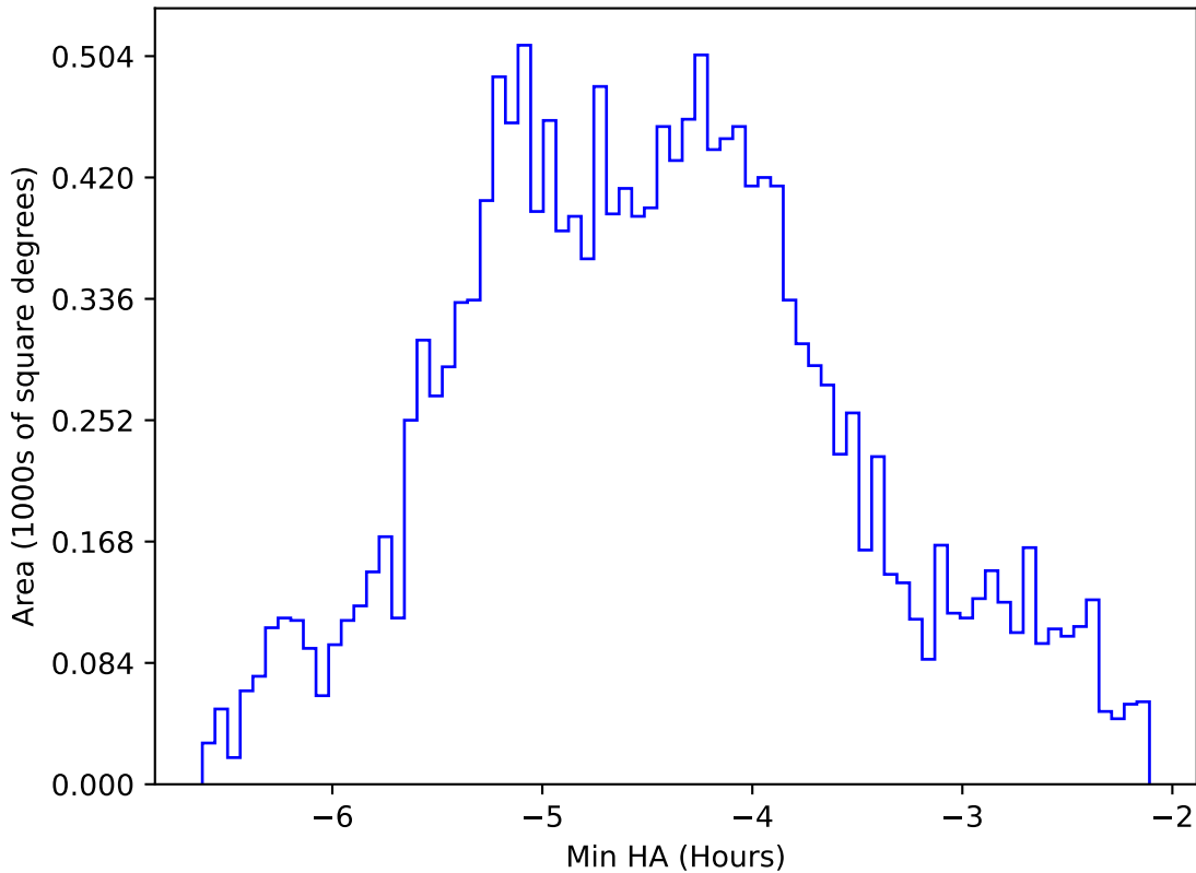
baseline_v3.2_10yrs WFD z band: Min HA
