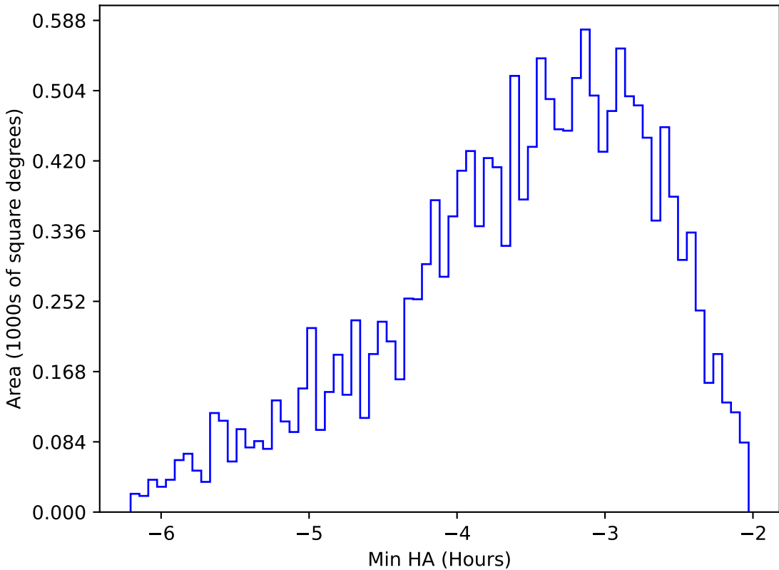
baseline_v3.2_10yrs WFD y band: Min HA
